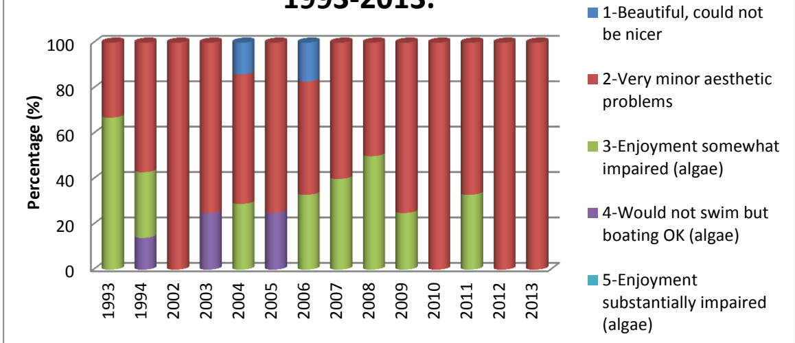
Figure 16. Van Vliet aesthetic value, 1993-2013.
